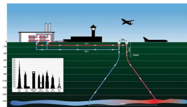
Schéma descriptif de l'installation géothermique d'ADP
